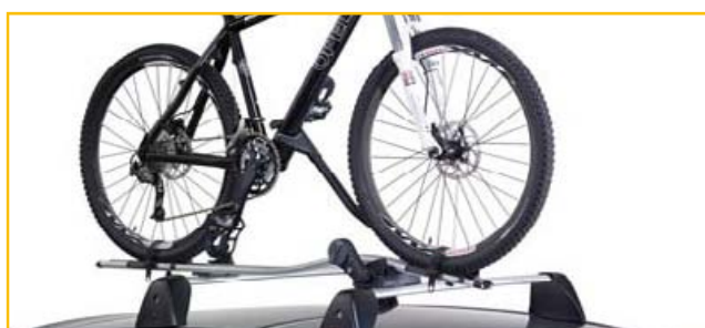
Uchwyt rowerowy Thule ProRide 591
